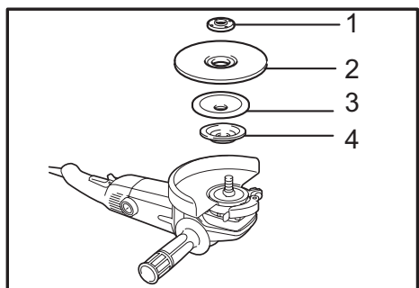
► 1. Contratuercas 2. Disco flexible 3. Plato de goma 4. Brida interior
