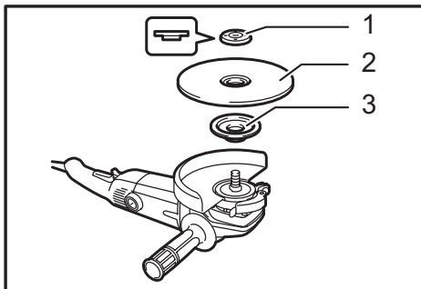
► 1. Contratuera 2. Disco de centro hundido/multidisco 3. Brida interior
